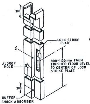
6A SIDE HUNG DOOR FRAME
